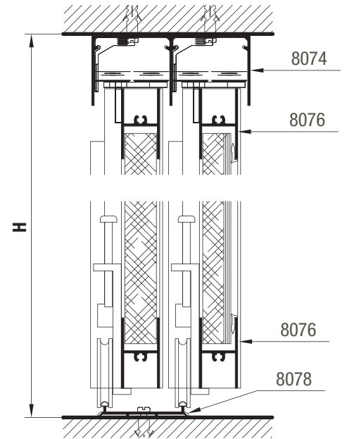
SECCION 4-5
