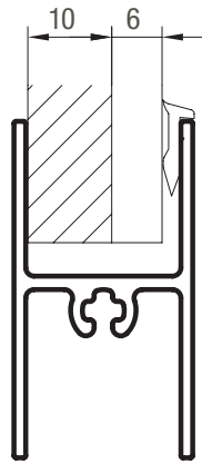
PLACA + ESPEJO
