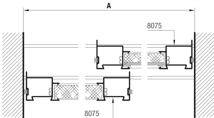
SECCION 1-2-3
